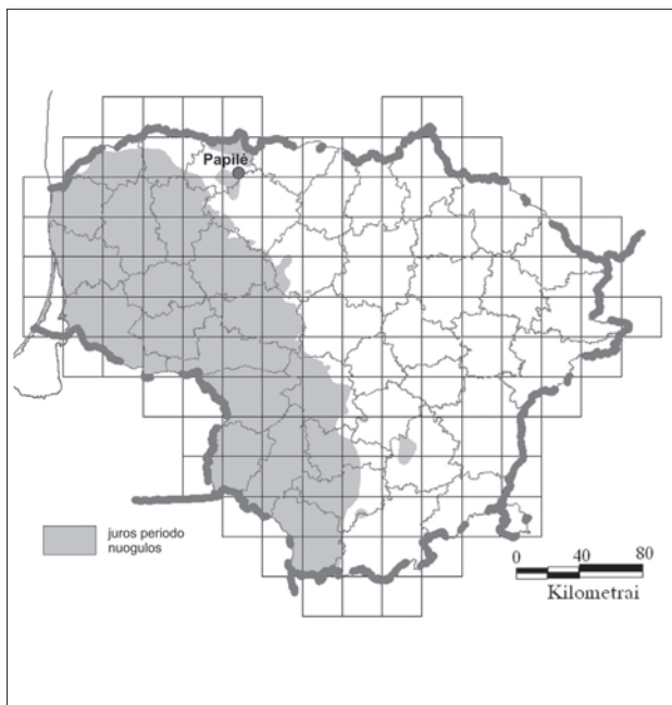
Juros uolienų paplitimo schema Lietuvoje
