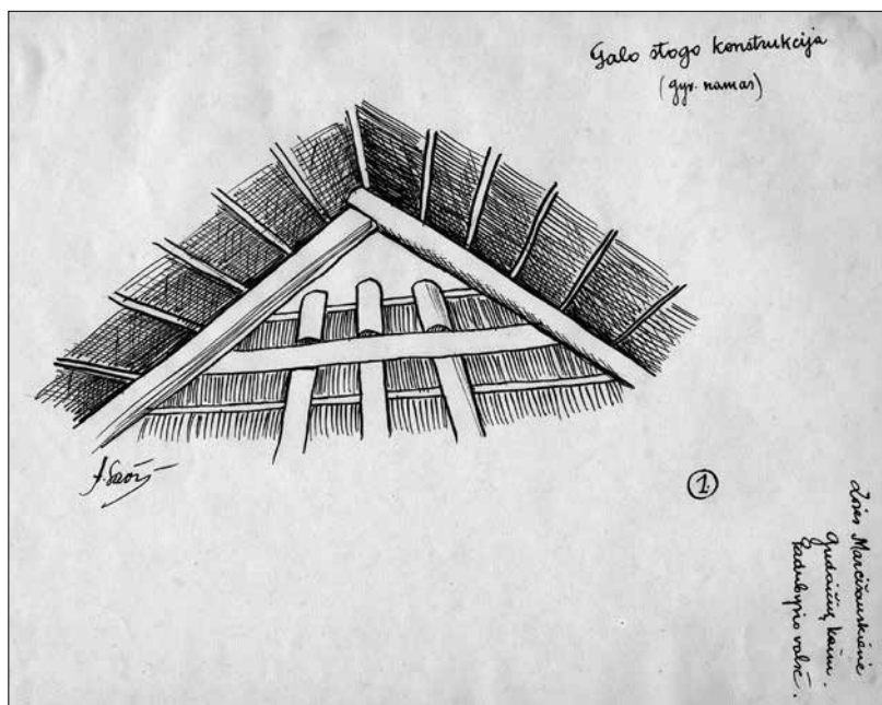
Gyvenamojo namo stogo konstrukcijos viršutinė dalis
